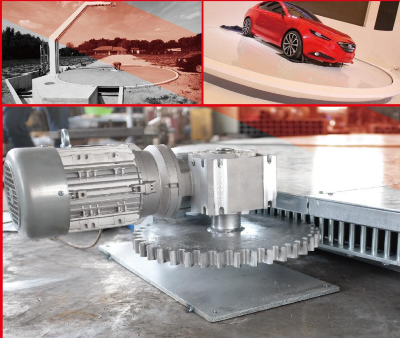
角度控制转台 / 升降旋转台 / 超薄销齿转台（83mm高）
